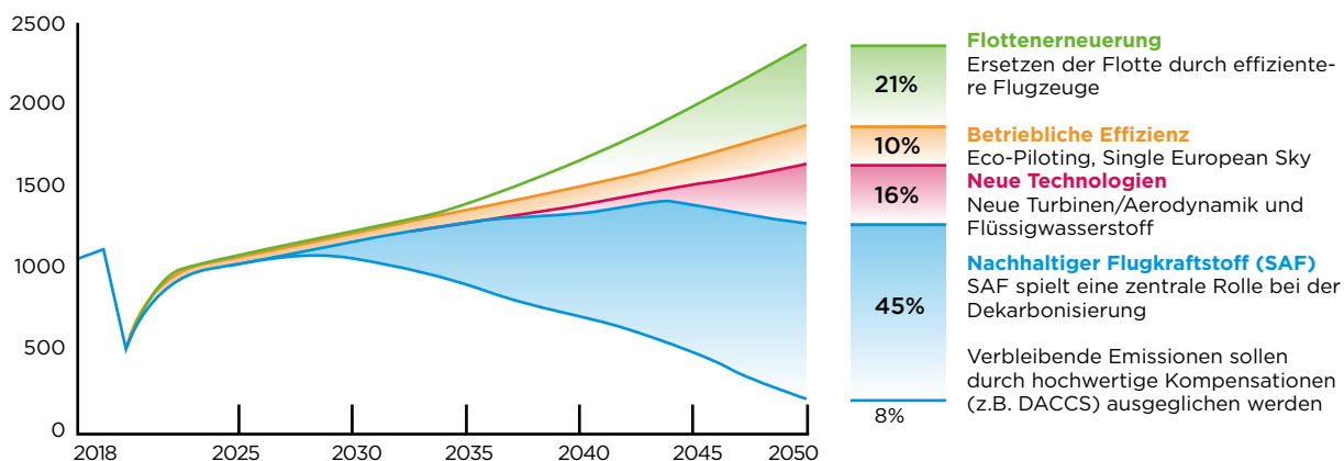
Zielpfad für CO 2 -Emissionen (gemäß Rat für die französische Luftfahrtforschung CORAC)
